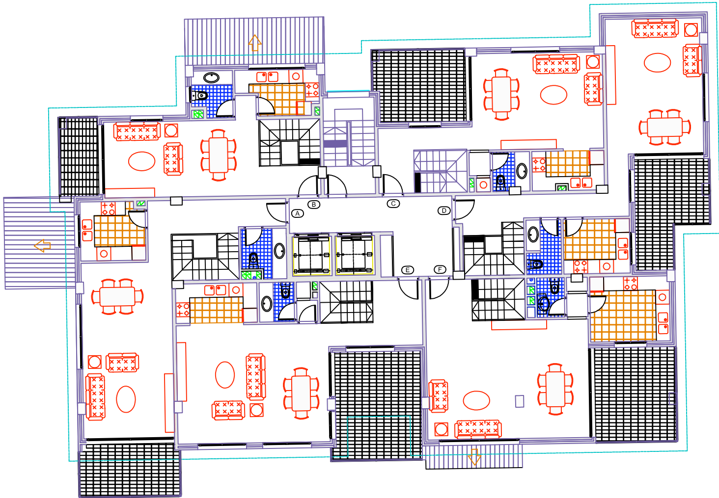
BLOQUE 2 - PLANTA PISO DUPLEX -
