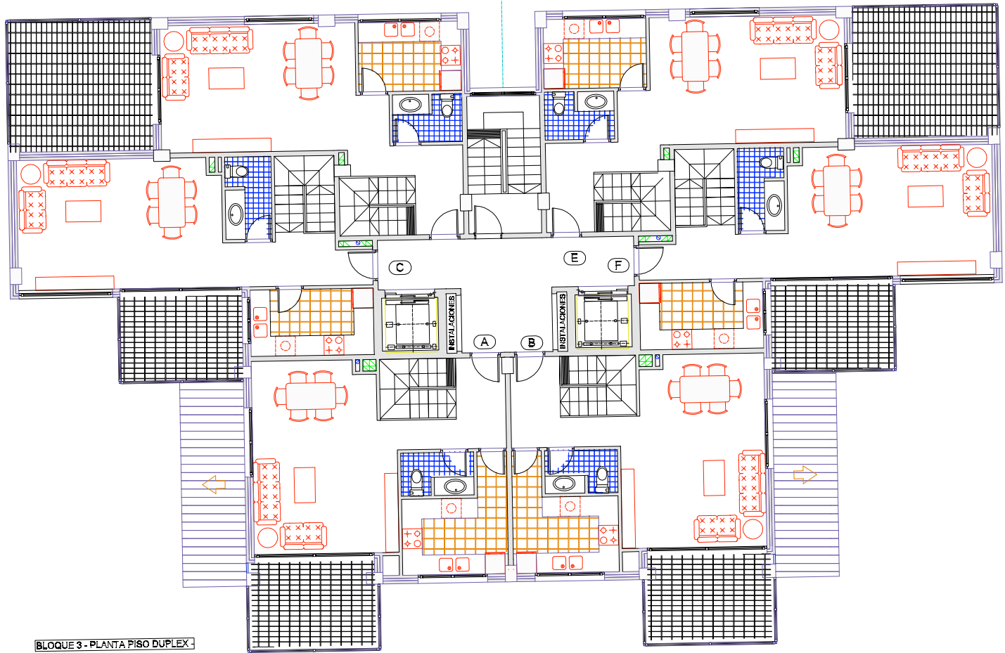
BLOQUE 3 - PLANTA PISO DUPLEX
